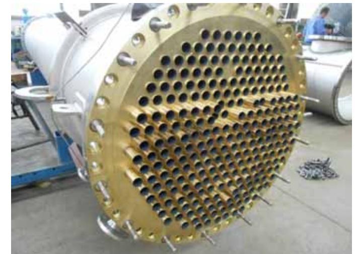
Wärmeaustauscher in verschiedenen Materialien wie z.B. Monel, Titan, Alu-Bronze, Graphit
