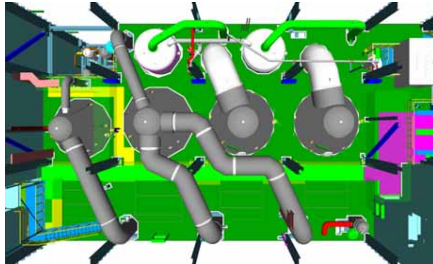
Brüdenrohrleitung Ø 2.600 mm
