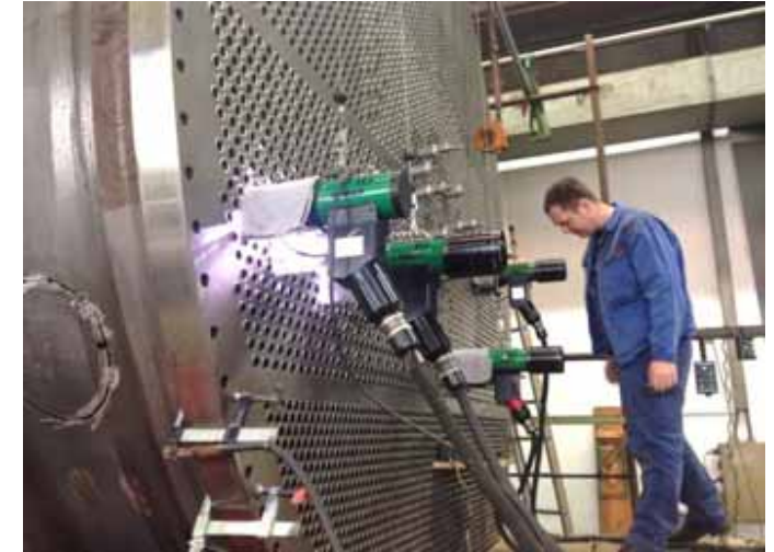
Fertigung und Montage (Niederlande) Seewasserkondensator Ø 3.650 mm, Gesamtlänge 10.000 mm, 40 t, 1.4462/P355GH
